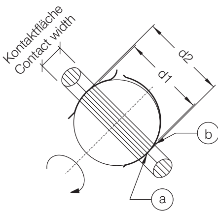
Detail A-A
